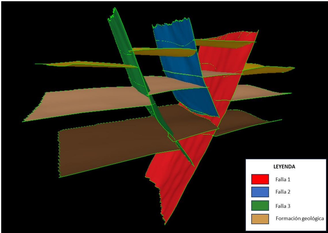
Figura 21. Modelo estructural
