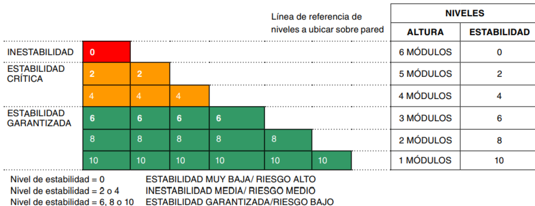
Grafico 1. Relación orientativa estabilidad/altura para apilados sobre pared de unidades de carga paletizadas
