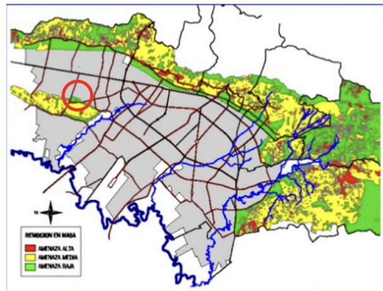
Mapa 2. Amenaza remoción en masa (derrumbe). Dentro de Círculo la UPZ 23, con una amenaza media de derrumbe debido a inclinación.
