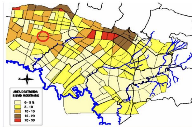
Mapa 1. Destrucción por sismo Moderado. Dentro de Círculo la UPZ 23, con un área proyectada de 5-10% de área destruida.
